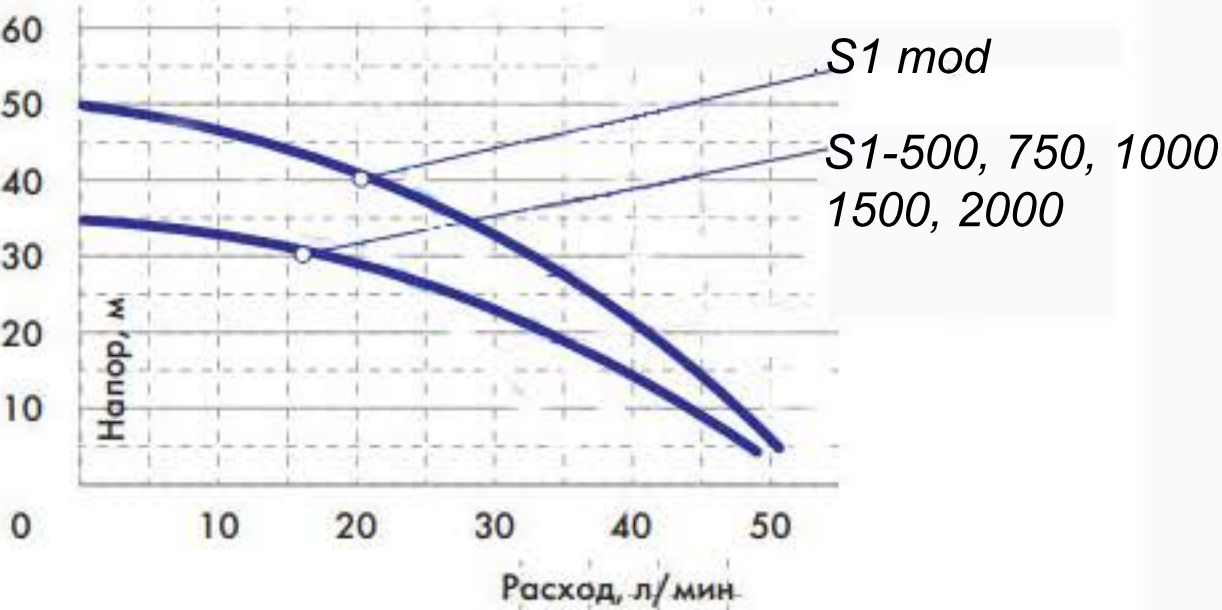
Гидравлические характеристики
