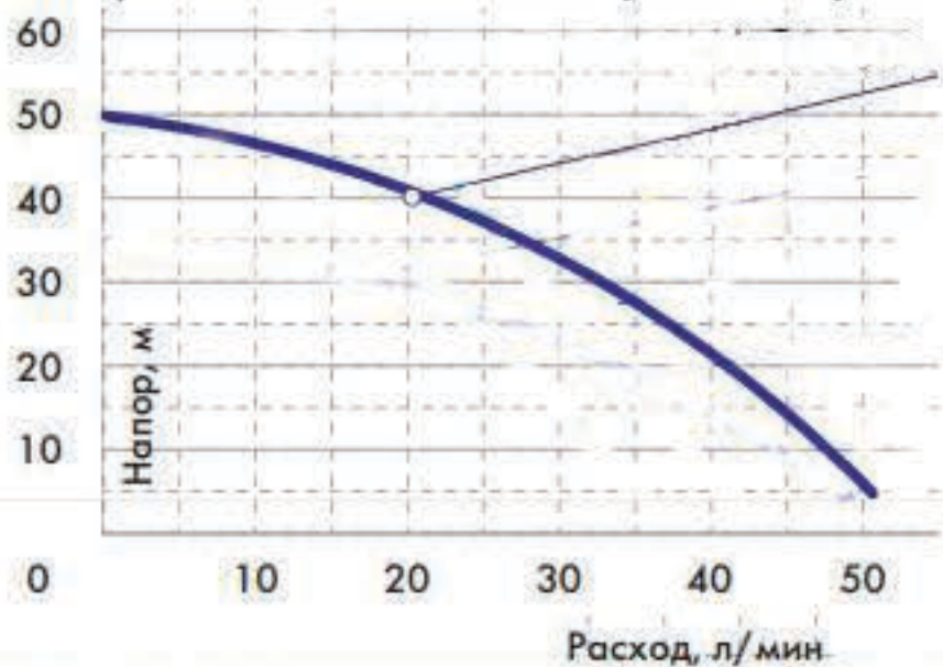
Гидравлические характеристики
