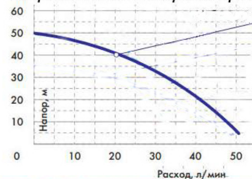
Гидравлические характеристики
